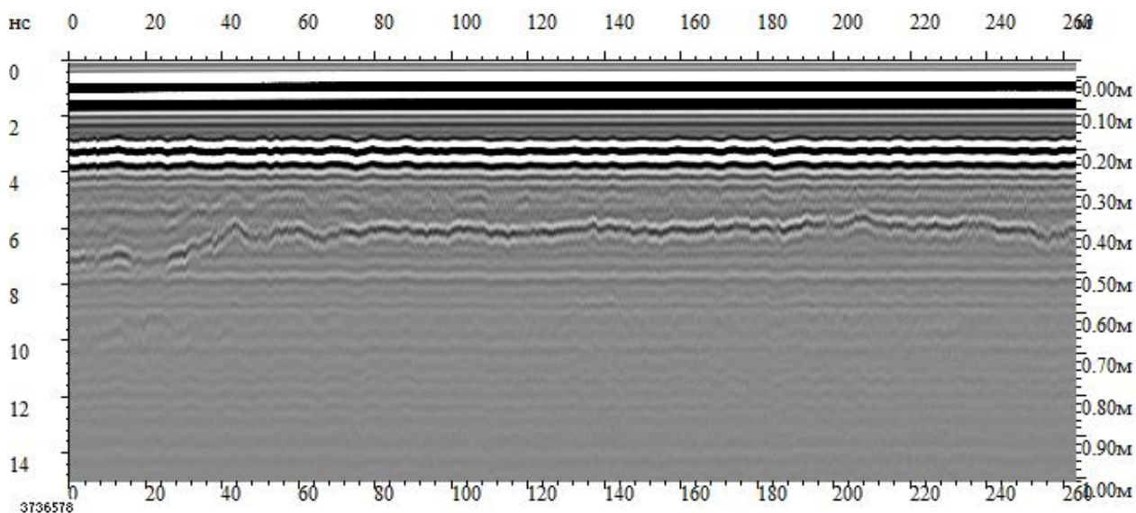
Рисунок Ж.1 – Исходная радарограмма продольного прохода (1700 МГц)
