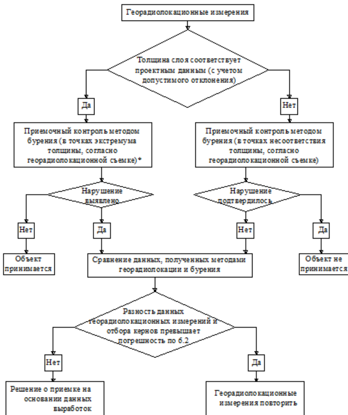
Рисунок А.2 – Алгоритм выполнения приемочного георадиолокационного контроля
