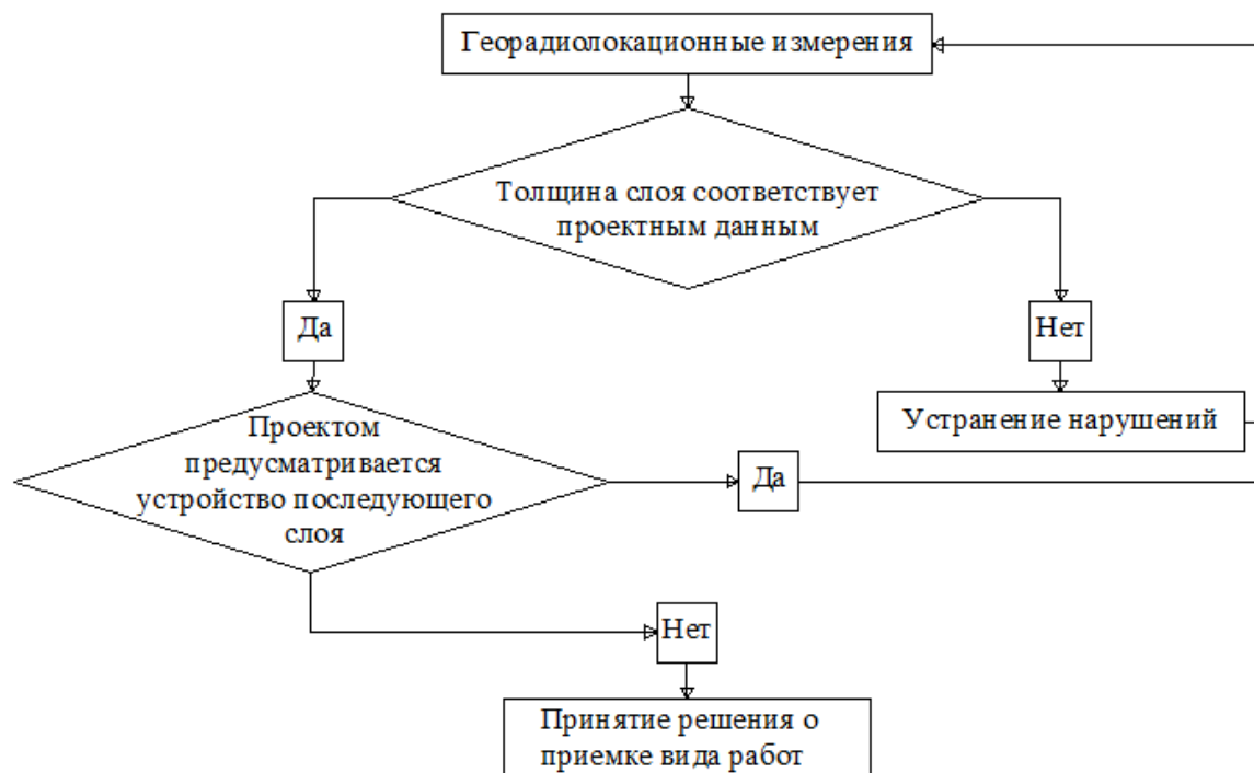
Рисунок А.1 – Алгоритм выполнения георадиолокационного операционного контроля
