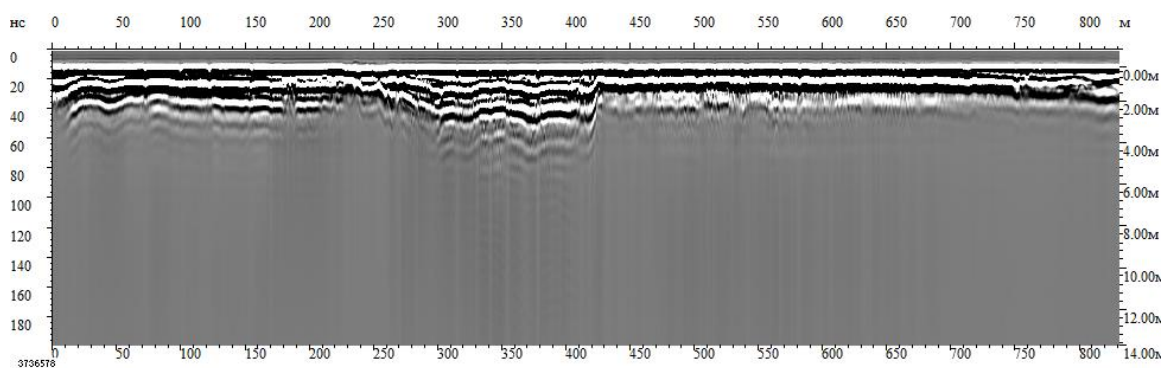
Рисунок Ж.3 – Исходная радарограмма продольного прохода (150 МГц)
