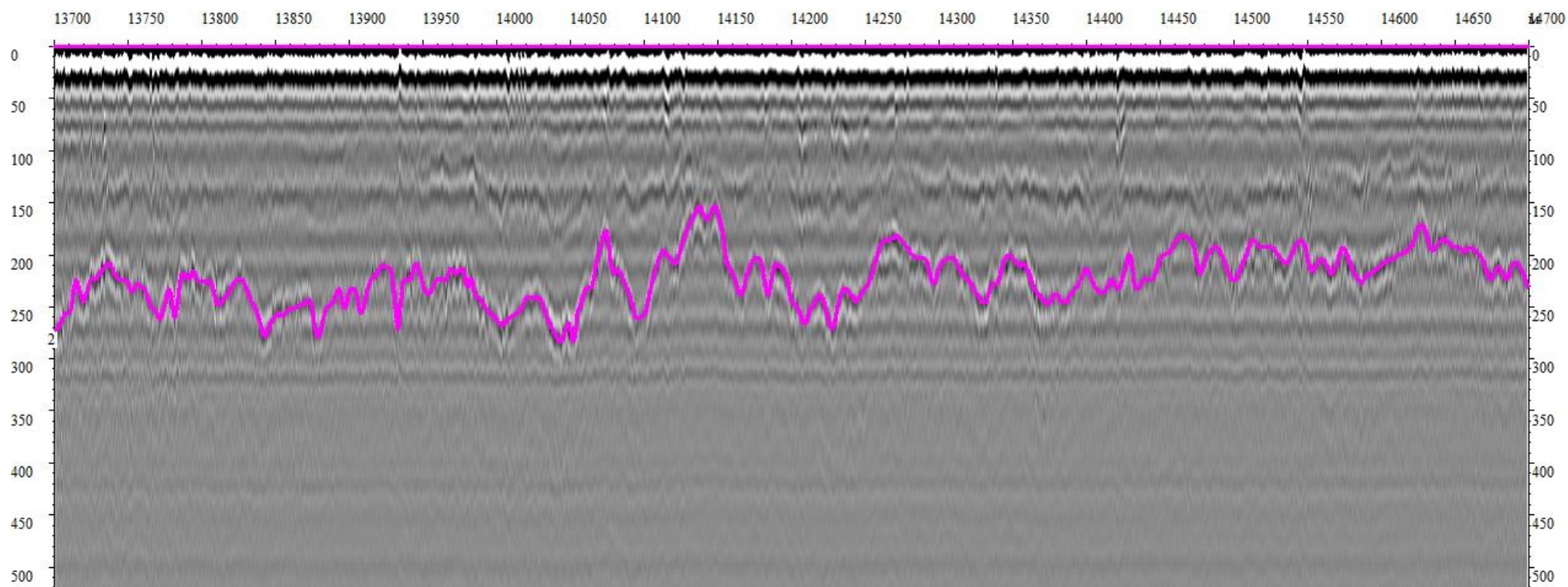
Е.1 Примеры оформления радарограмм продольных профилей
