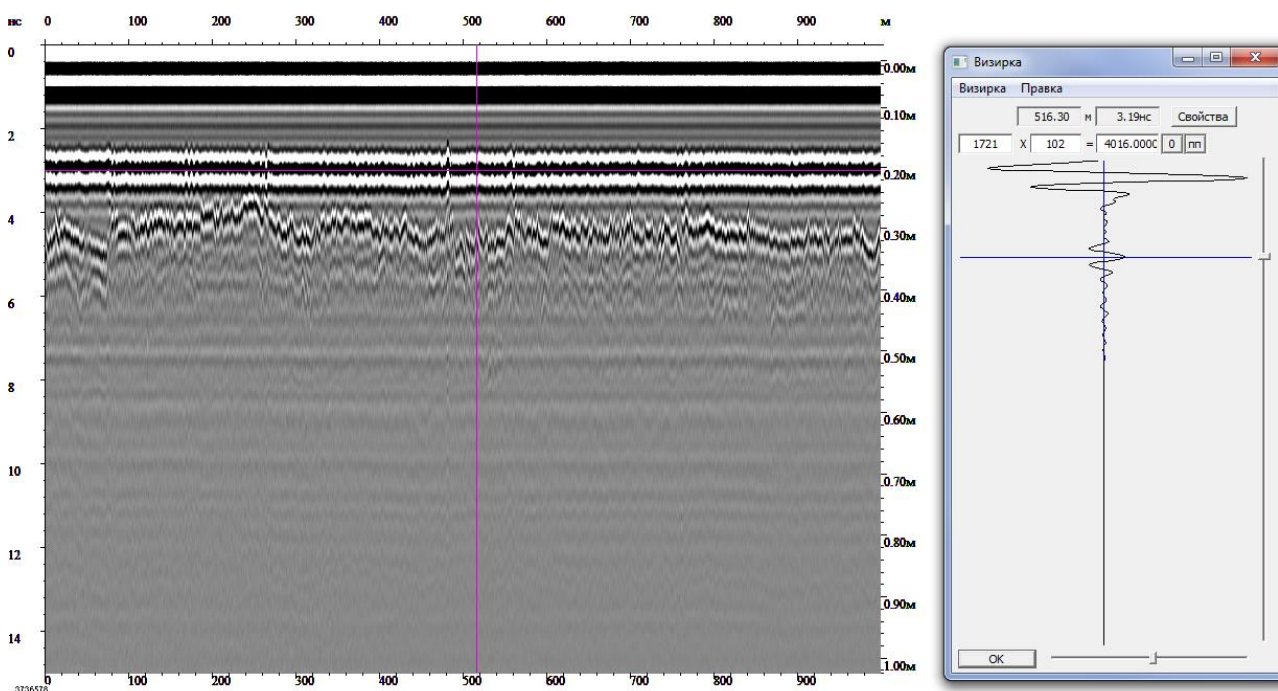
Рисунок Д.1 – Пример смещения вертикальной шкалы глубин
