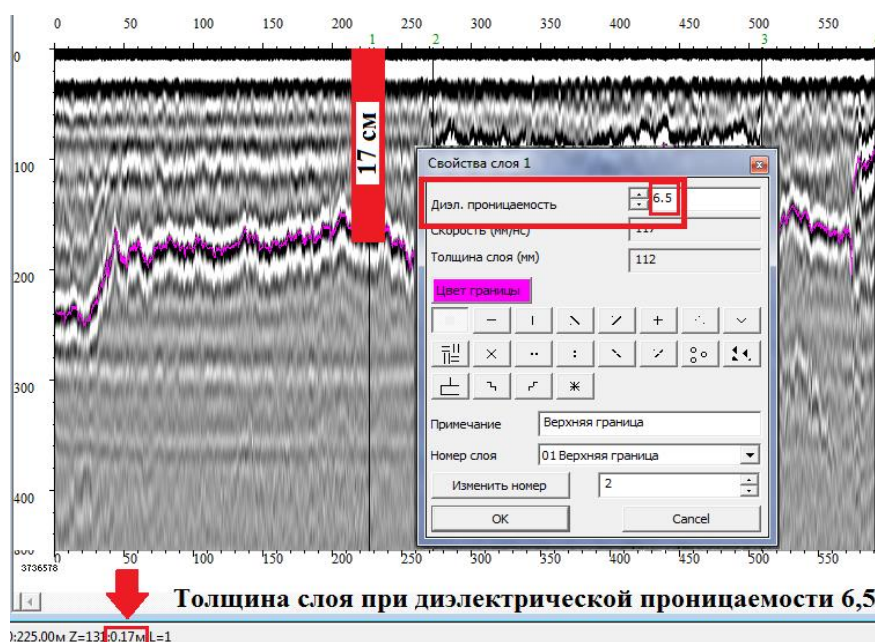
Рисунок 4 – Толщина слоя после корректировки диэлектрической проницаемости
