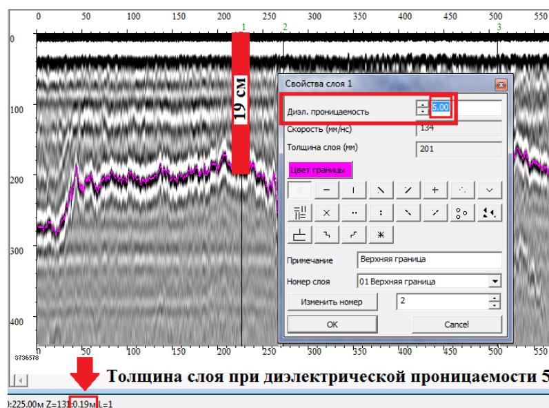
Рисунок 3 – Толщина слоя до корректировки диэлектрической проницаемости
