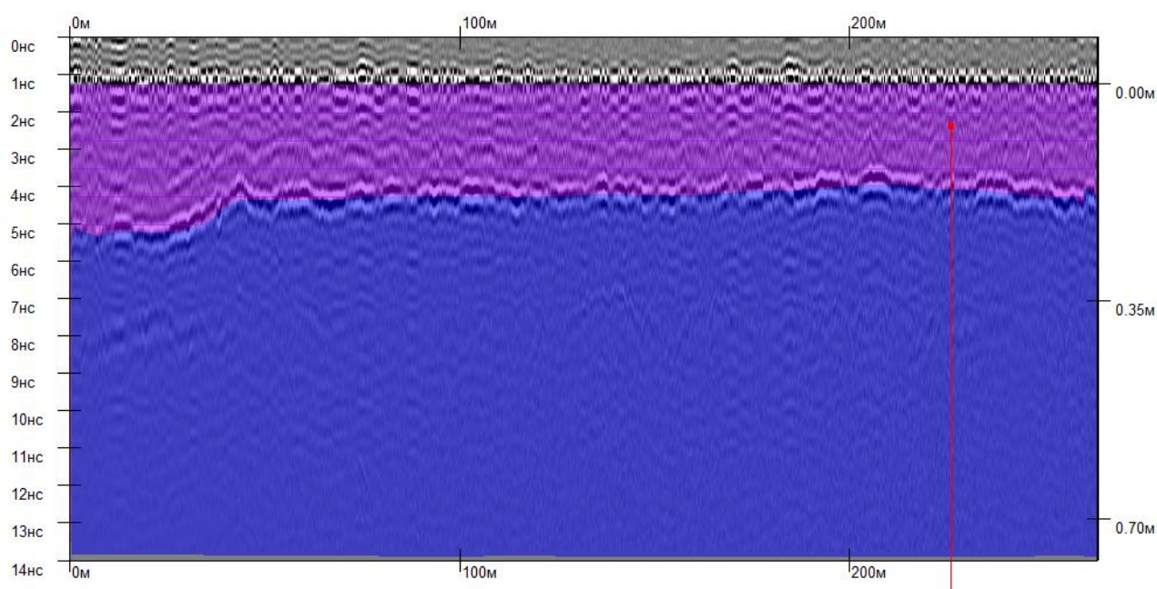
Рисунок Ж.2 – Радарограмма продольного прохода после обработки (1700 МГц)
