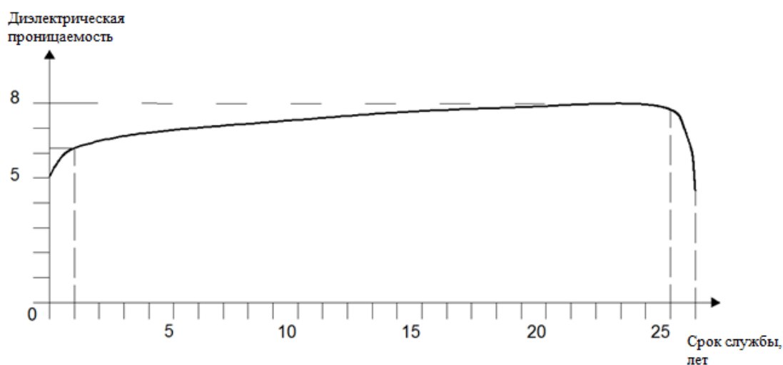
Рисунок 1 – Зависимость диэлектрической проницаемости слоев асфальтобетона от их возраста
